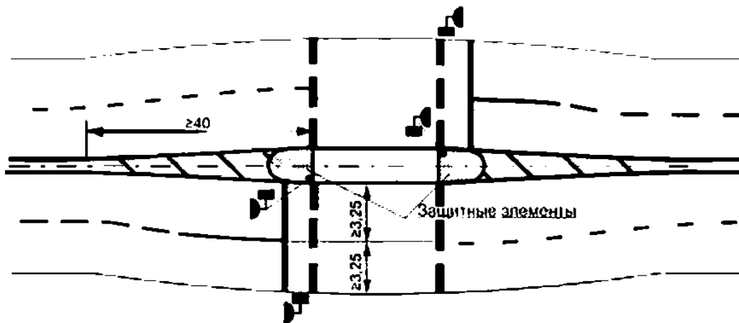
Рисунок Б.6 — Устройство островка безопасности
